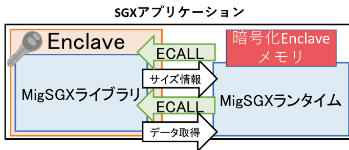
図 4 Enclave の状態データの取得
