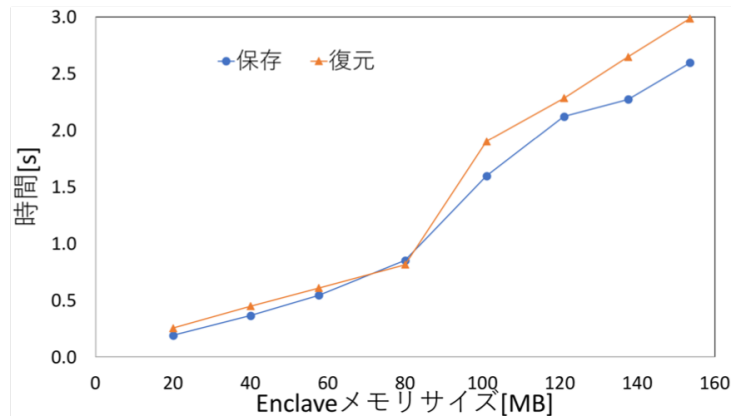
図 7 保存・復元の性能
