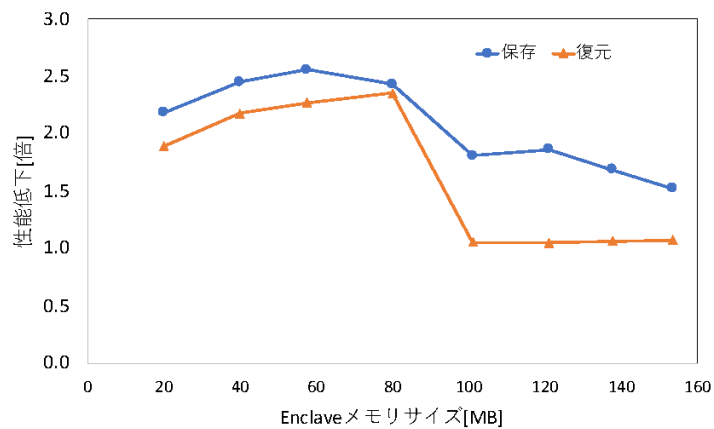
図 8 暗号化オーバーヘッド
