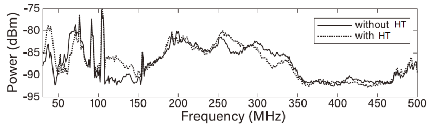
図 14 HT の有無による電子機器の不要放射スペクトル変化
