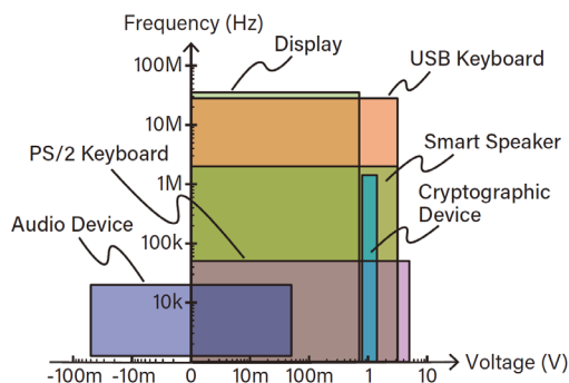
図 11 機器内部信号の電圧・周波数分布
