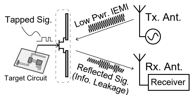
図5 機器内に実装されたハードウェアトロージャンと電磁波照射を併用した情報窃盗の原理
