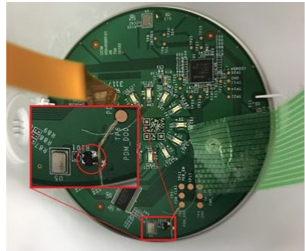
図 4 スマートスピーカ内部に実装されたハードウェアトロージャン（丸囲み内の素子）
