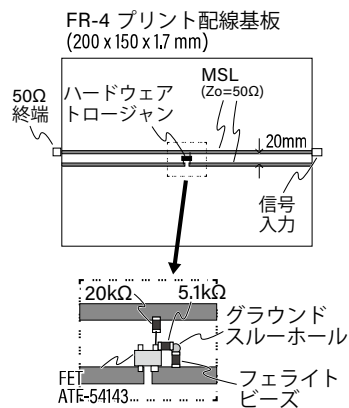
図6 機器とハードウェアトロージャンの単純化モデル
