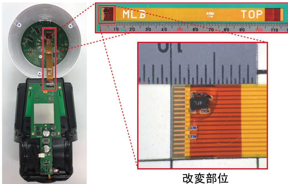
図 13 スマートスピーカへの回路改変攻撃例
