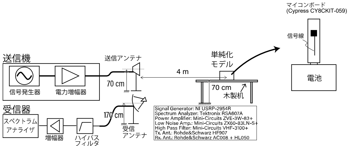
図9 AI/IoT 機器の単純化モデルを用いた回路改変無しターゲットに対する情報漏えい評価システム
