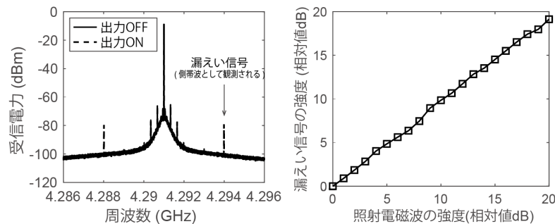
図10 単純化モデルへの電磁波照射により観測された漏えい信号および照射強度に対する漏えい強度の変化
