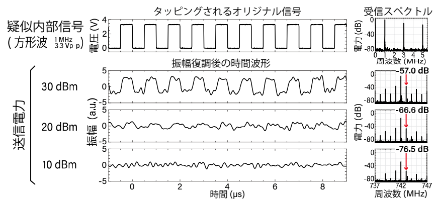
図8 評価結果 (オリジナル信号形状復元の忠実度評価および、情報を含むスペクトル強度による漏えい有無の評価)
