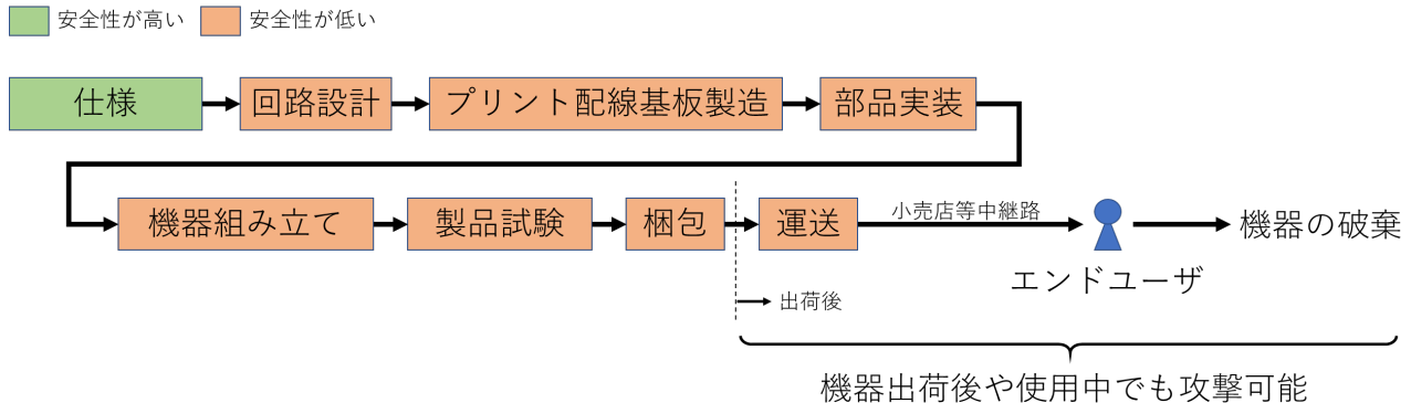
図3 IC周辺回路へハードウェアトロージャンが実装されるタイミング
