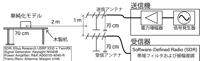
図7 評価システムおよびその配置
