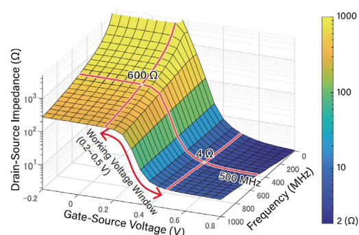
図 12 HEMT ATF-54143 の電氣的特性
