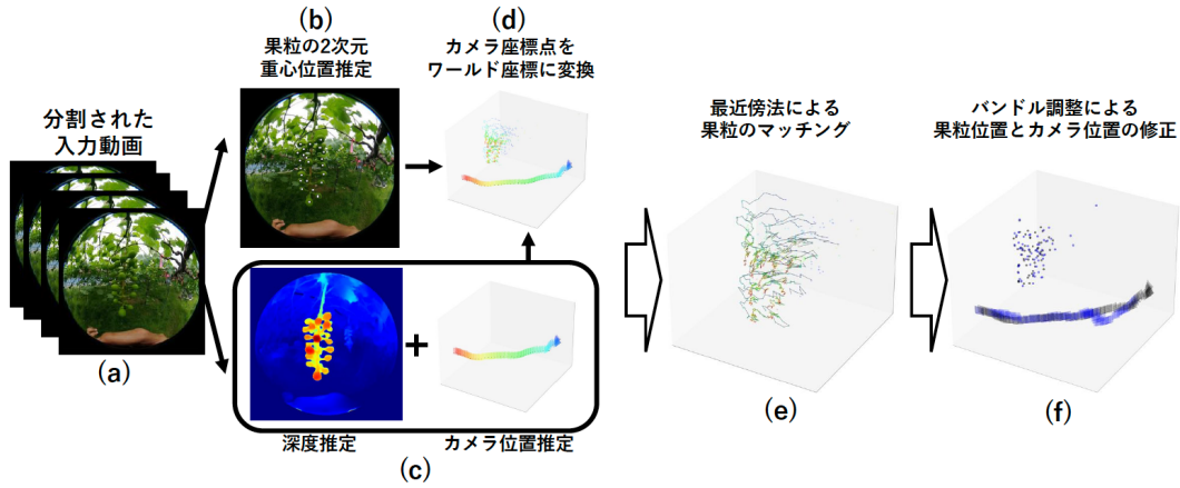
図 5: ブドウ房の部分的な果粒配置推定の流れ
