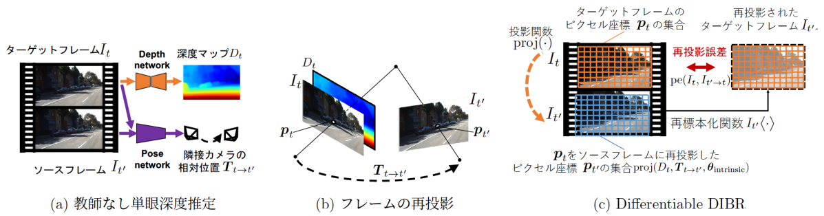
図 2: Differentiable DIBR を用いる教師なし単眼深度推定
