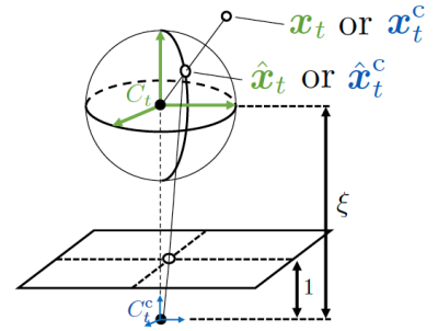
図3 : Unified Omnidirectional Camera Model ( C_t の座標系は緑色、 C_{ct} は青色で記載)
