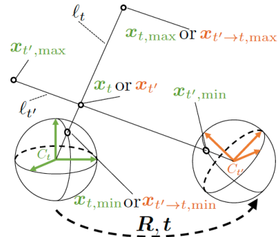
図4: Scale-Aware Constraint ( C_t の座標系は緑色, C_{t'} はオレンジ色で記載)
